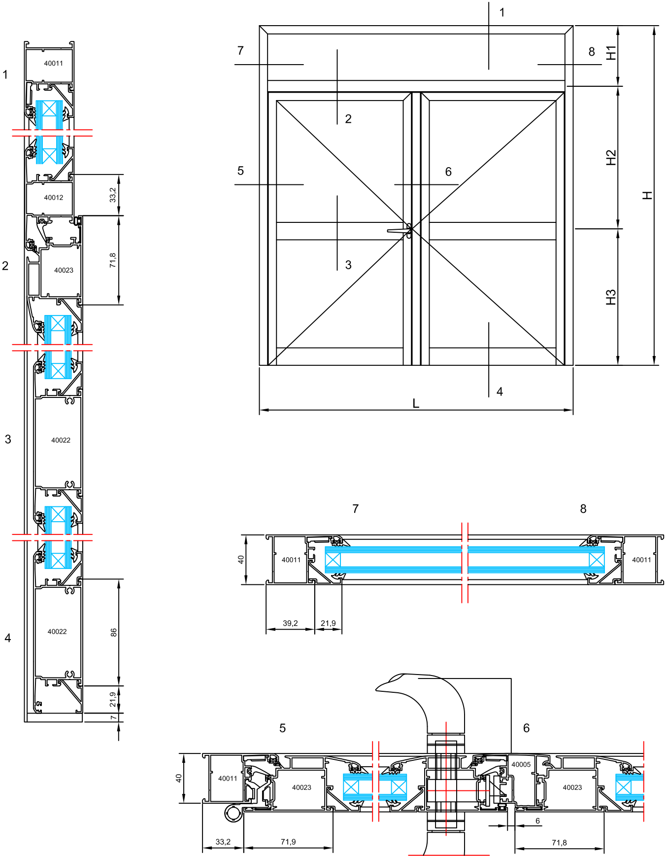
Escala Sección 1:3
