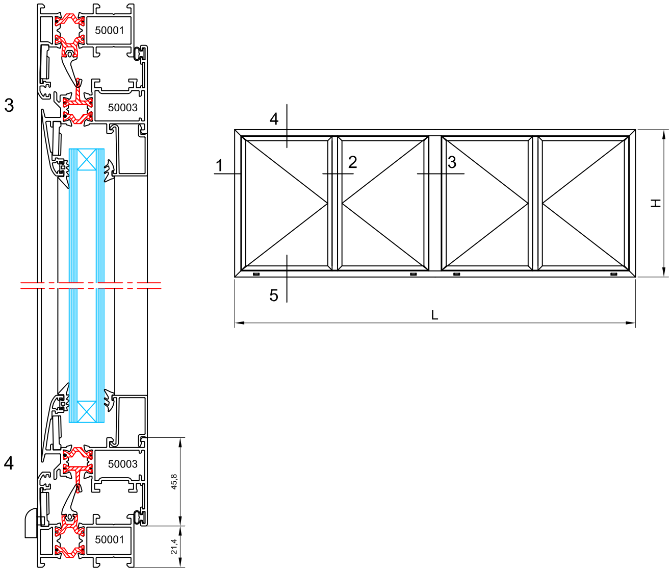
Escala Sección 1:2
