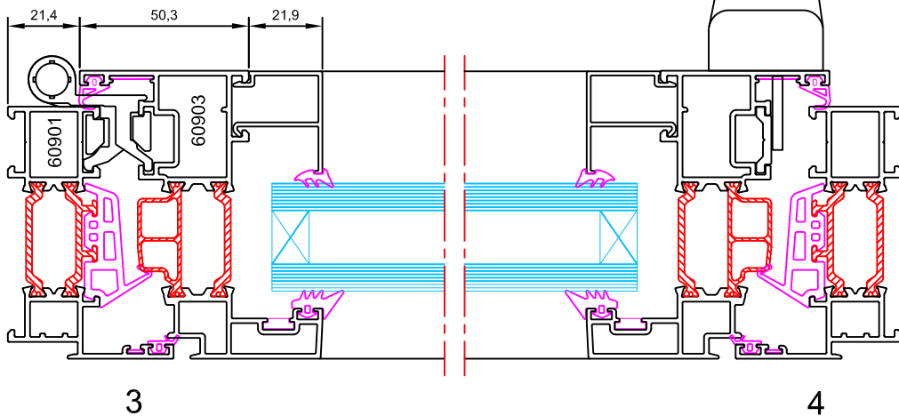
Escala Sección 1:2
