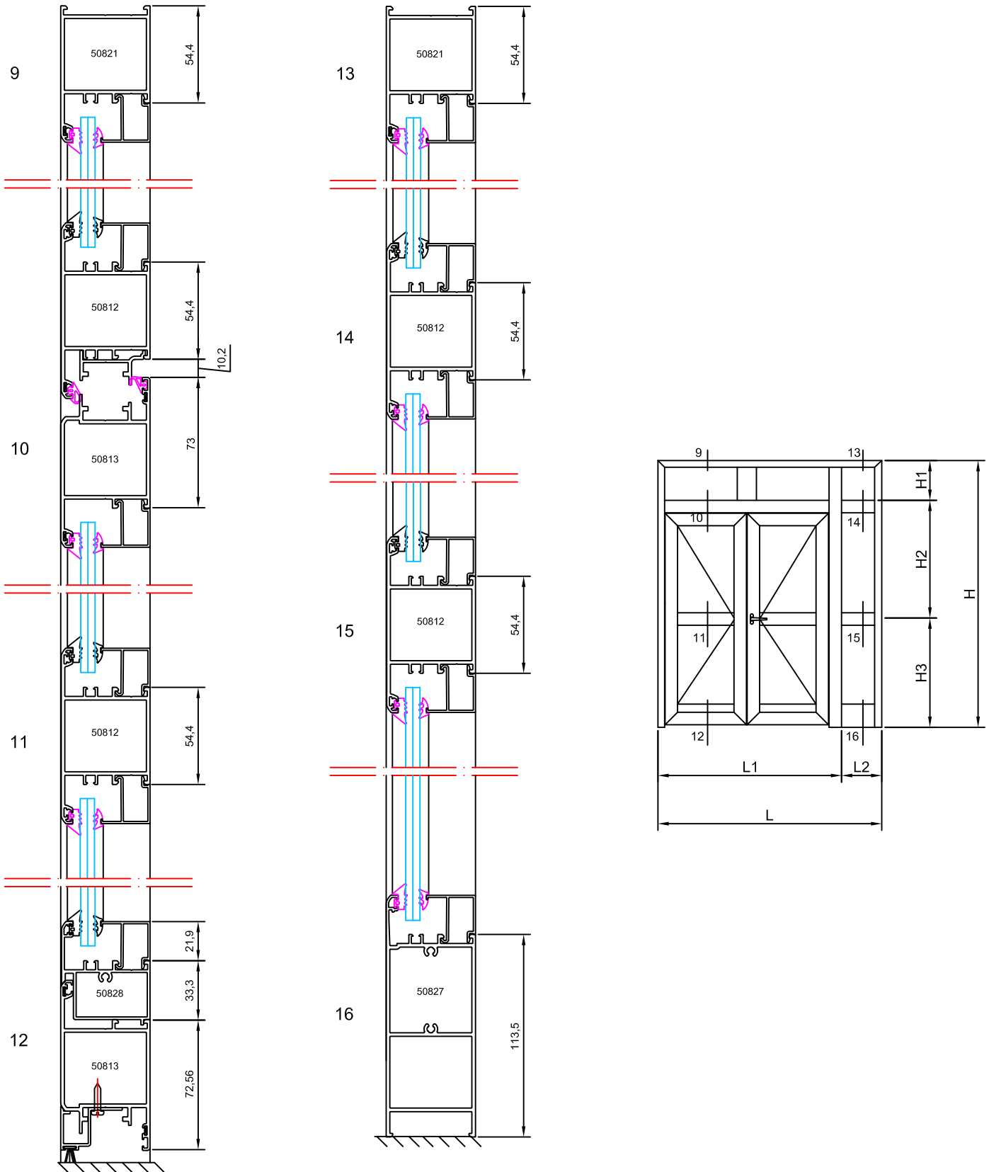
Escala Sección 1:3
