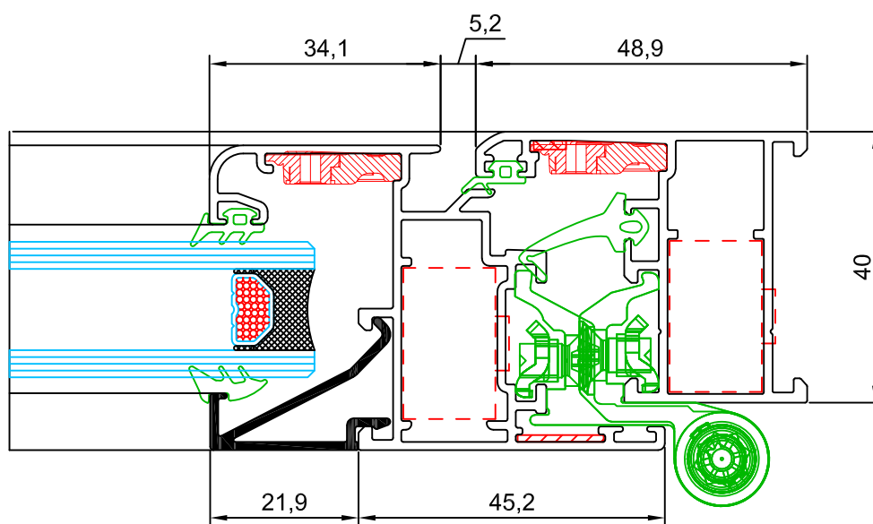
sección 3
