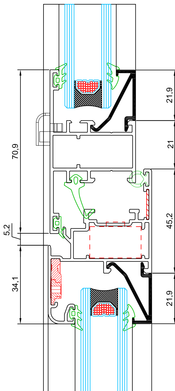
sección 6
