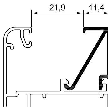
10002 junquillo 11,4 mm
