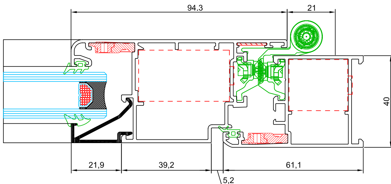
sección 13
