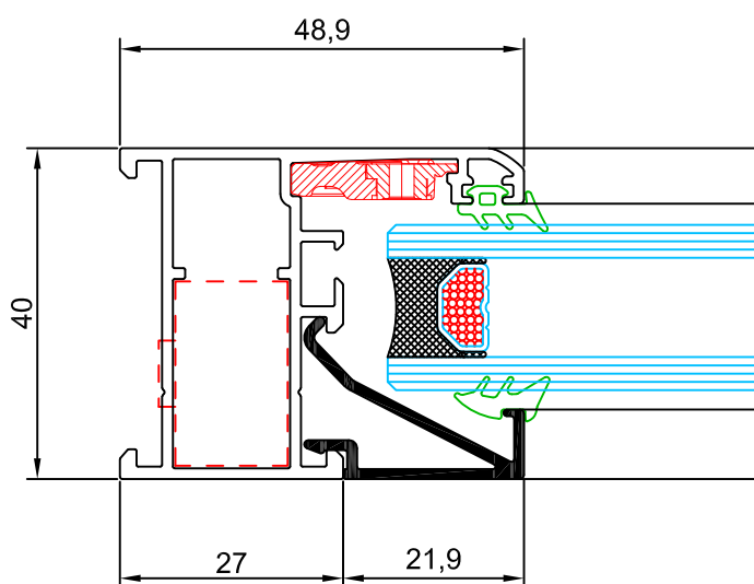
sección 1
