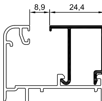
10006 junquillo 24,4 mm
