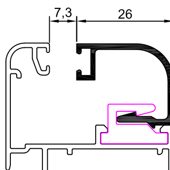
12004 junquillo 26 mm
