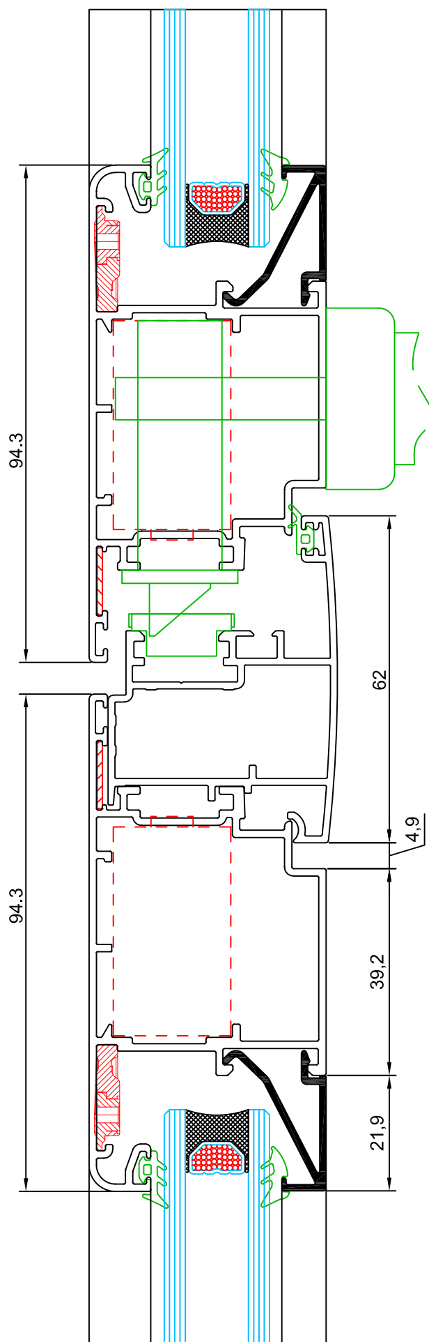
sección 16
