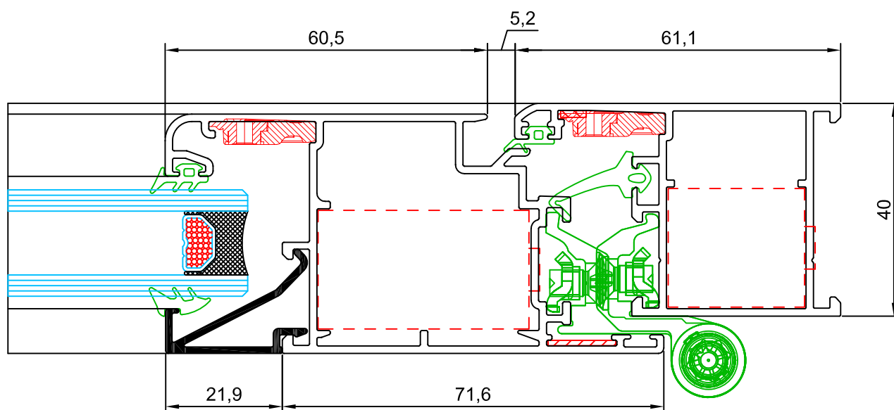
sección 7
