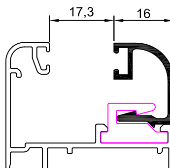
12002 junquillo 16 mm
