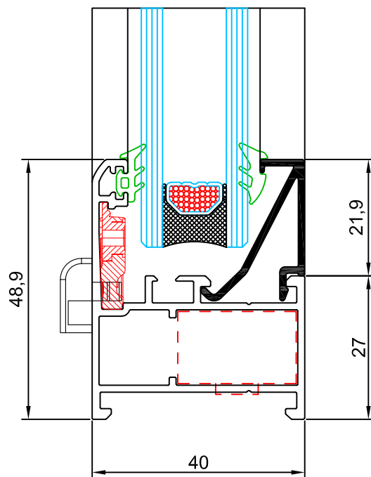
sección 2
