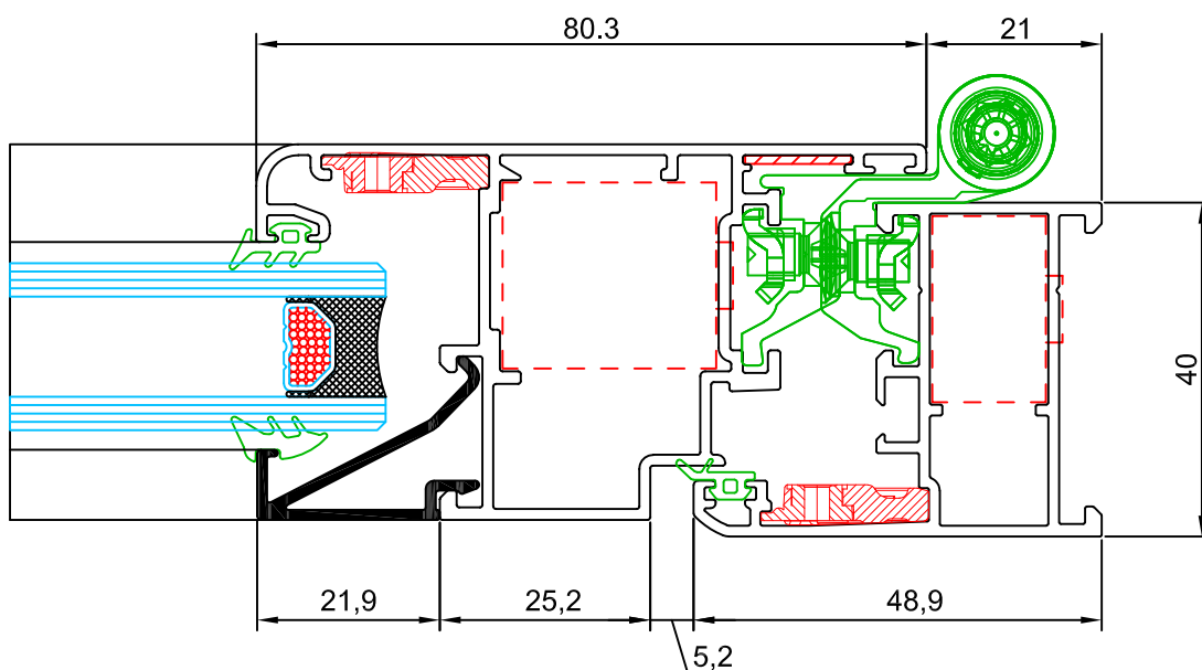
sección 12
