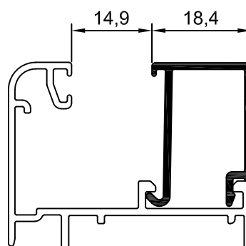
10004 junquillo 18,4 mm
