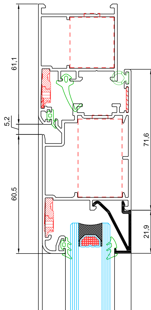
sección 8
