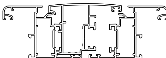
Escala 1:2
