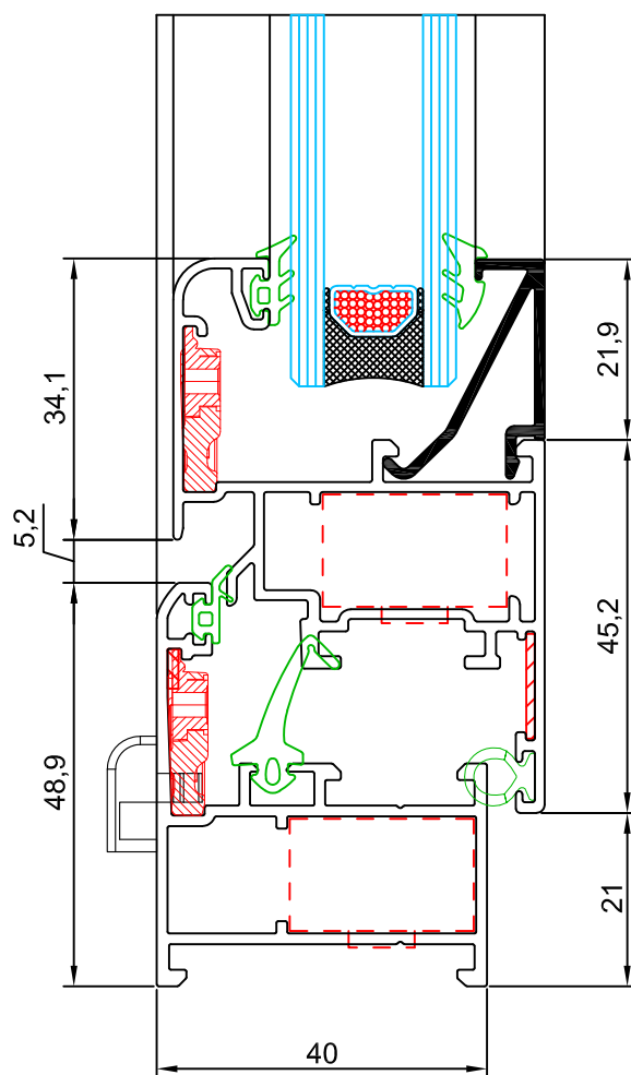
sección 4
